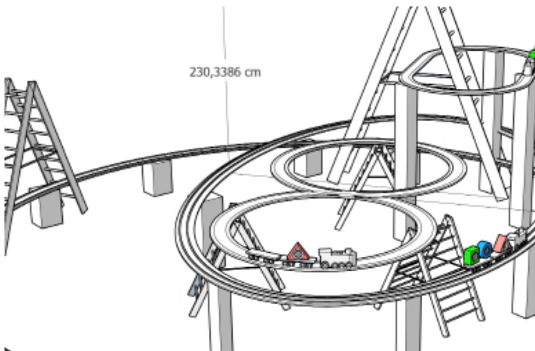
étude de volume pour le circuit géant (sept 2020)
